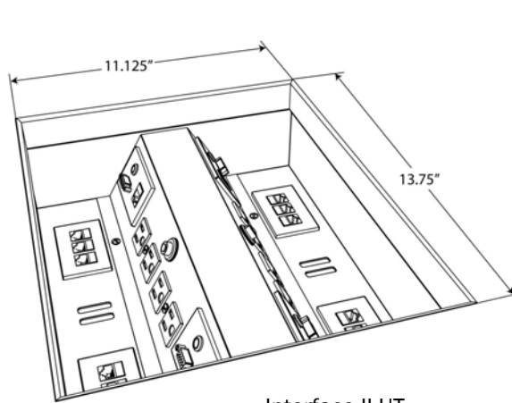
Interface II UT
