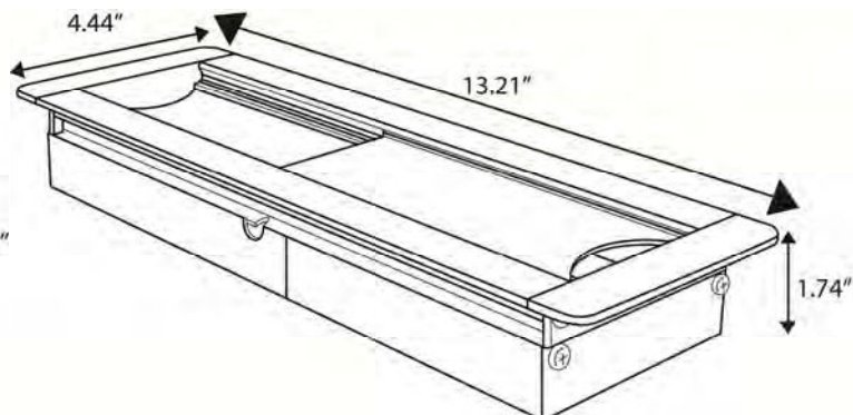
MARINA MINI GROMMET
